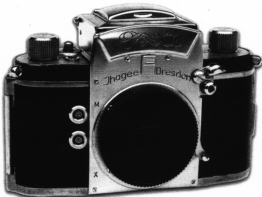
Diese Kamera entspricht im Grunde dem oben abgebildeten Modell. Interessant ist jedoch die bis dato in der einschlägigen Literatur nicht aufgeführte Gravurvariante der Blitzbuchsen.
