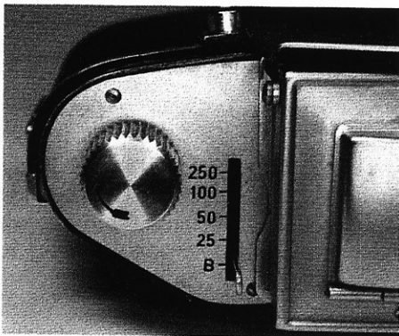
Sowohl die Exa Varex als auch die erste Serienfertigung der Exa (V. 1.1) besaßen als kürzeste Verschlusszeit die 1/250 s. Alle nachfolgenden Kameras erhielten dann die 1/150 s, die bequem über einen Schalter zu bedienen sind.
