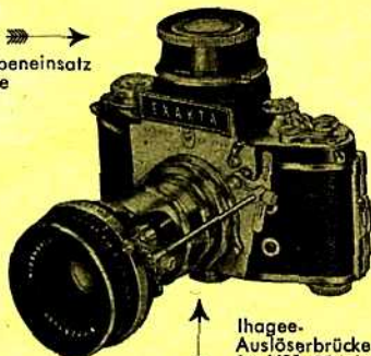
EXAKTA Varex
