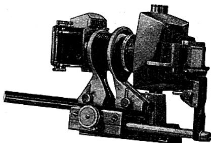
EXAKTA Varex mit Dia-Kopiervorsatz am Balgnaheinstellgerät
