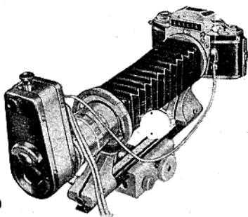
Reprogerät mit Beleuchtungs- einrichtung
