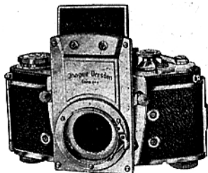
EXAKTA Varex mit Lichtmeßeinrichtung
