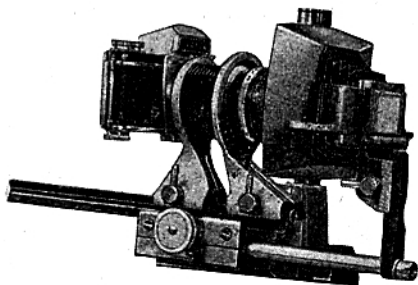
EXAKTA Varex mit Dia-Kopiervorsatz am Balgennaheinstellgerät
