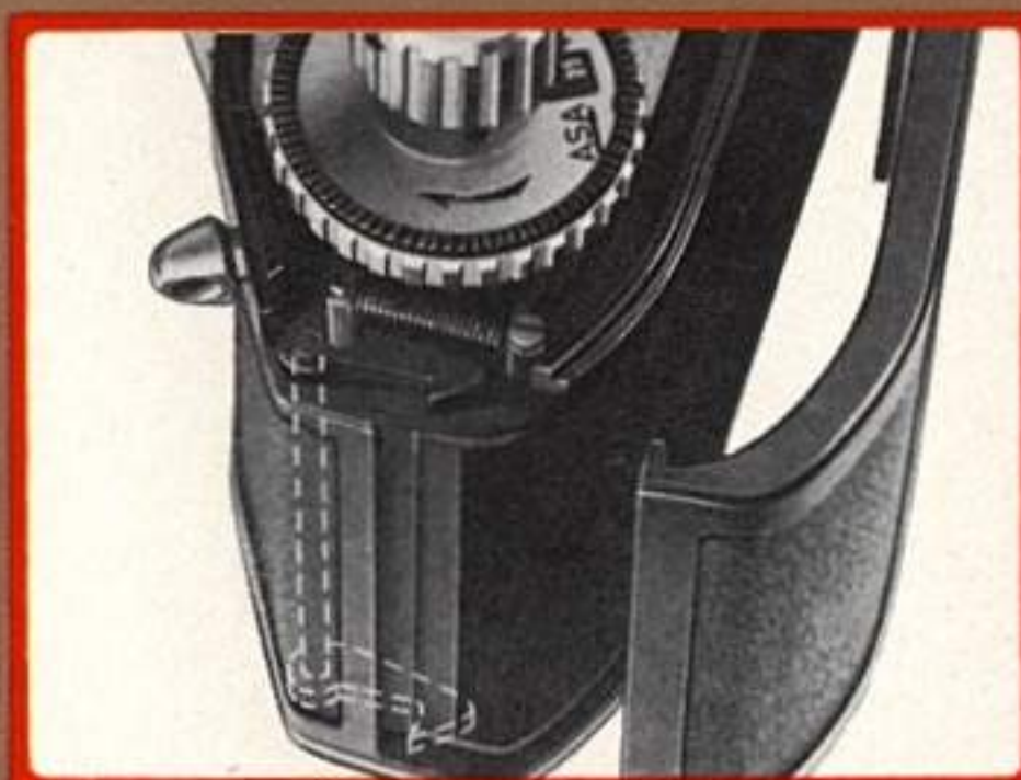
Neue Anordnung der Rückwandverriegelung (Rückwand aus verwindungs- freiem Spritzguß)
