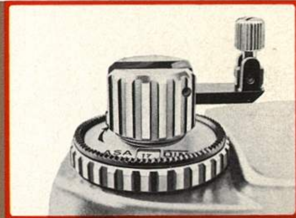
Selbstausröser mit Funktionsstop
