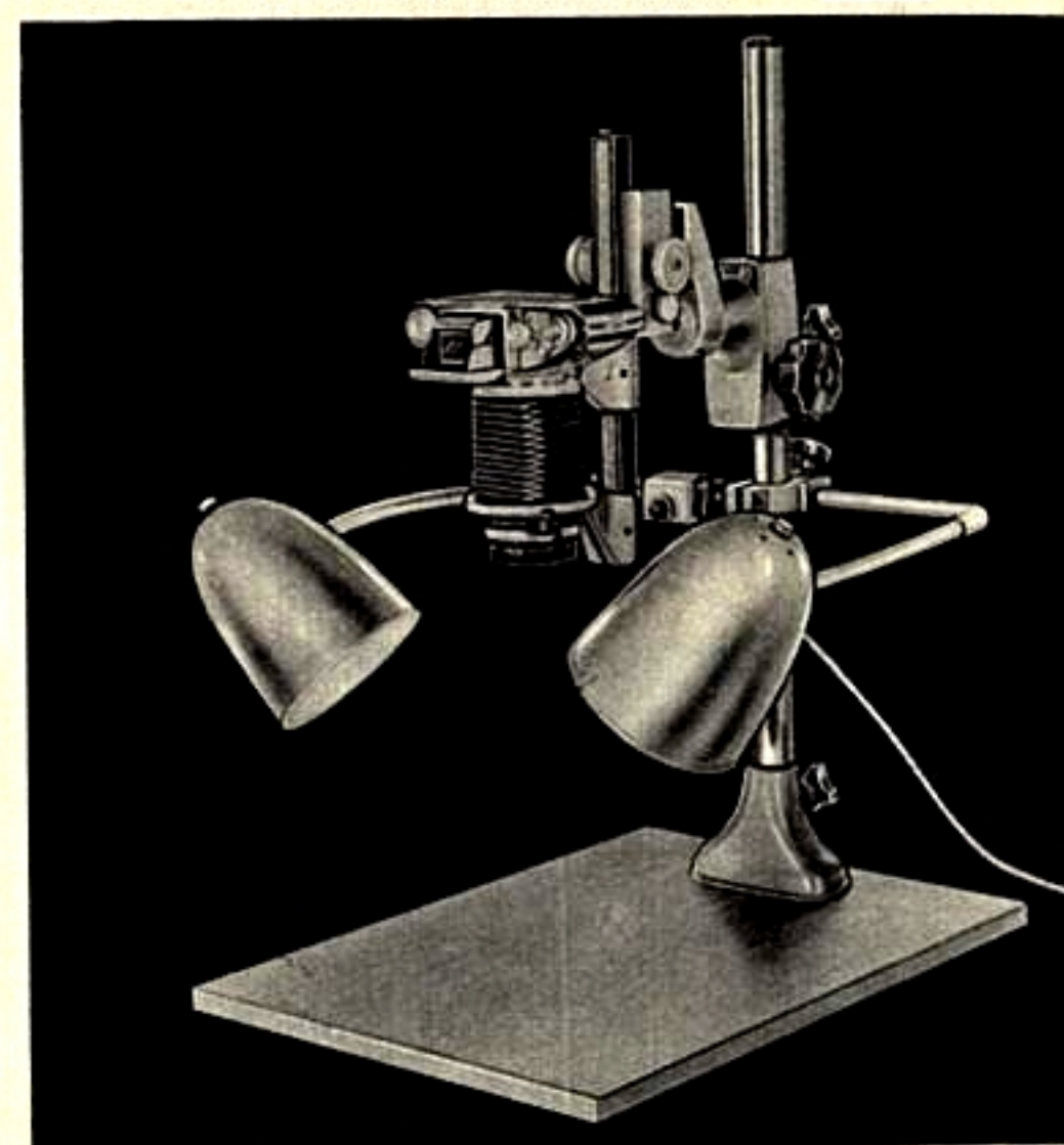
Reprokészülék megvilágítóberendezéssel
